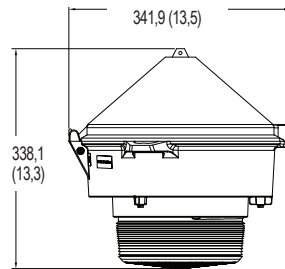
Montage sur montant incliné à 25° — Réflecteur
