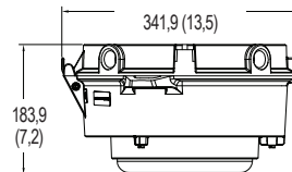
Montage sur montant incliné à 90° — Diffuseur
