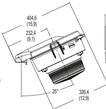
Montage plafond ou mural — Réflecteur
