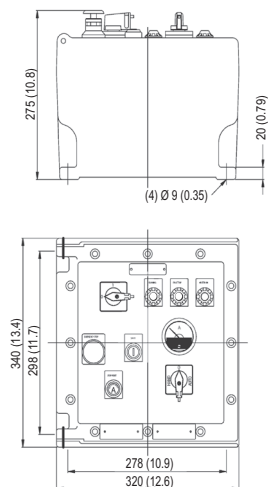
Taille 3 : CF30B
