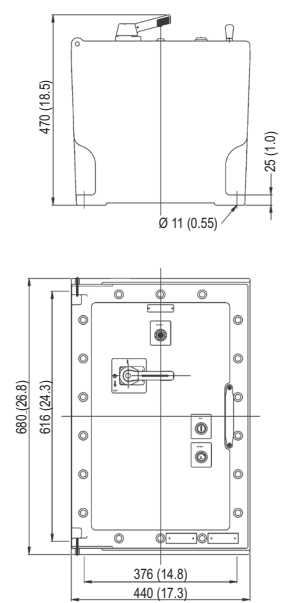
Taille 9 : CF60B
