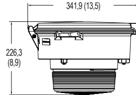
Montage conique suspendu — Réflecteur
