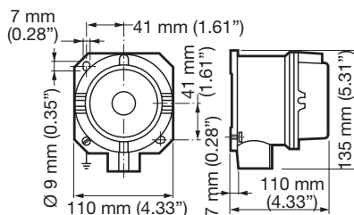
BR1d (2 Fonctions)
