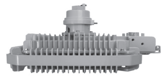
BHLP 24 K, 30 K, 38 K lumens avec option de suspension à montage rapide.
