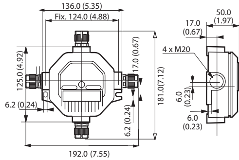
BJe1 avec entrée de câble pour câbles non armés
