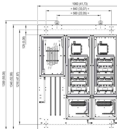
Vue intérieure
