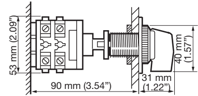
Commutateur montage fond de boîte
