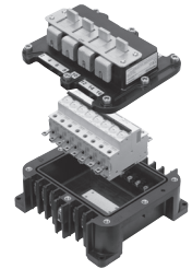
8 M Modulaires — Vue éclatée
