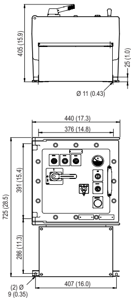
Taille 8 : CF50B + JBe47
