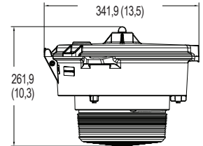
Montage plafond — Réfracteur
