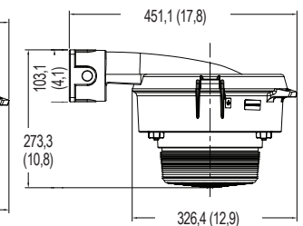
Montage mural — Réflecteur
