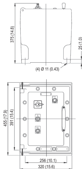
Taille 9 : CF60B
