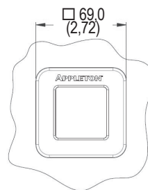
Fenêtre pour ampèremètre
