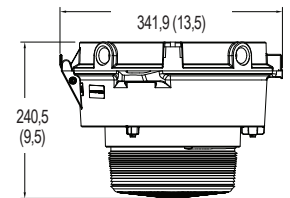
Montage sur montant incliné à 90° — Réfracteur
