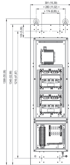
Vue intérieure
