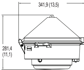
Montage sur montant incliné à 25° — Diffuseur
