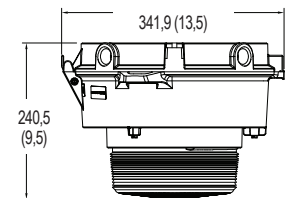
Montage sur montant incliné à 90° — Réflecteur
