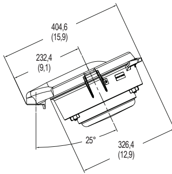
Montage plafond ou mural — Diffuseur
