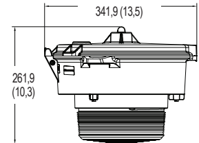
Montage plafond — Réflecteur
