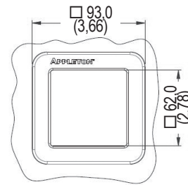
Fenêtre pour voltmètres
