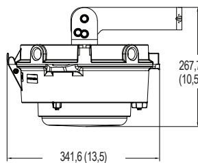
Montage plafond ou mural — Diffuseur
