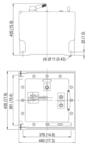
Taille 7 : CF50B
