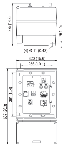
Taille 10 : CF60B + JBe55
