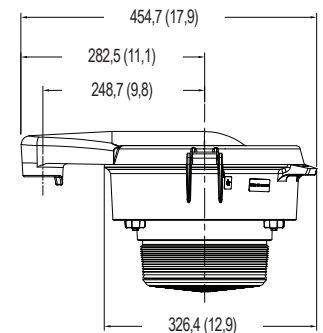
Montage mural — Réfracteur
