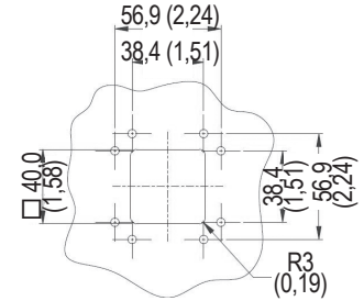
Informations sur le perçage
