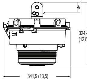
Montage plafond ou mural — Réfracteur
