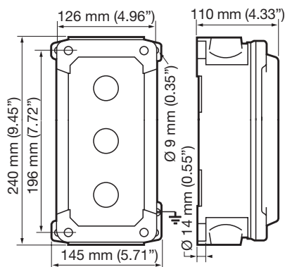
CF2D (3-4 Fonctions)
