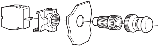
Bouton poussoir sur panneau
