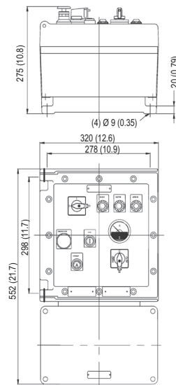
Taille 4 : CF30B + CAe2
