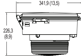
Montage conique suspendu — Réfracteur
