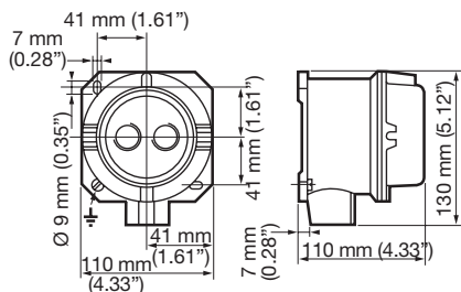
CF2D (2 Fonctions)
