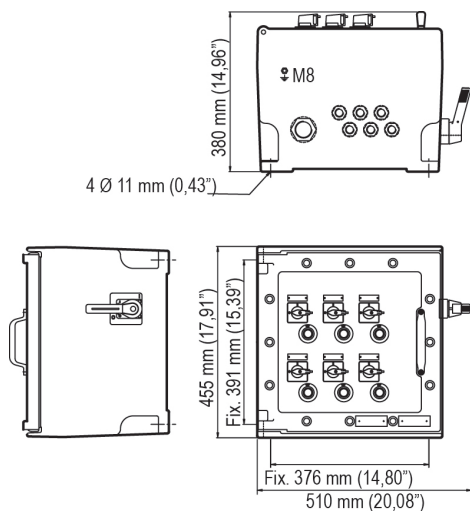
Schéma E
