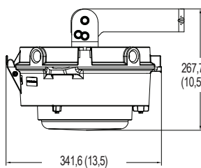
Montage plafond ou mural — Diffuseur
