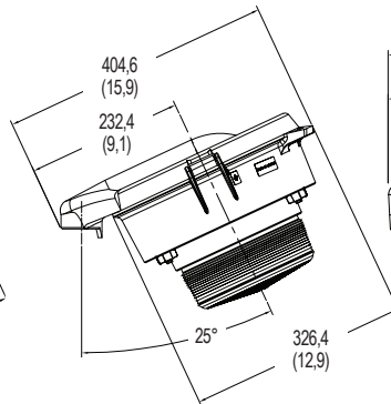
Montage plafond ou mural — Réfracteur
