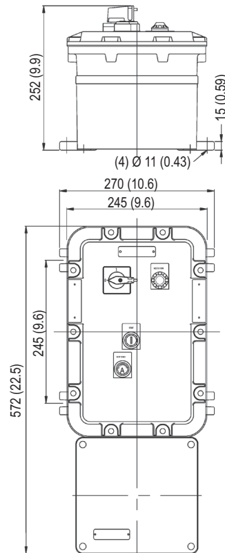
Taille 2 : CF20B + CAe1
