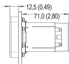
AC Ampèremètre — 72 mm x 72 mm (2,83 po x 2,83 po)
