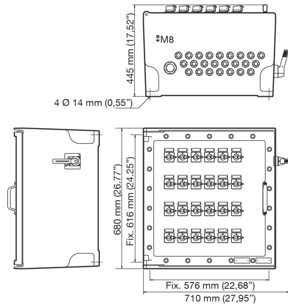
Schéma D
