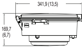
Montage conique suspendu — Diffuseur
