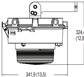
Montage plafond ou mural — Réflecteur
