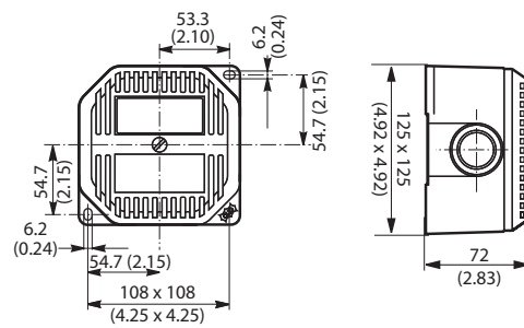
BJe2 avec entrée de câble pour câbles armés
