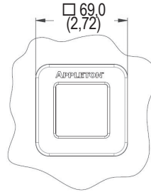
Fenêtre pour voltmètres
