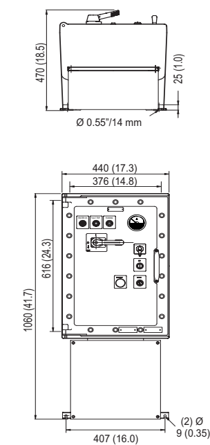
Taille 10 : CF60B + JBe55
