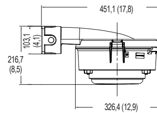
Montage mural — Diffuseur
